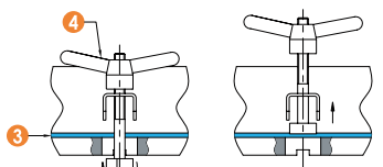
detail of unhooking/detail des Auslösung
